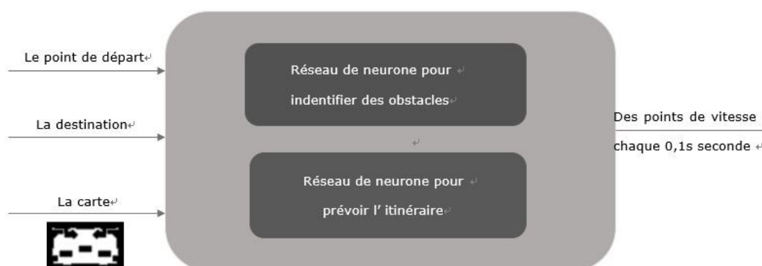
Figure 23 : Structure de combinaison des deux réseaux de neurones
