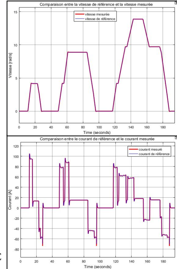
Figure 12. consignes en courant et en vitesse associées au cycle de conduite ECE
