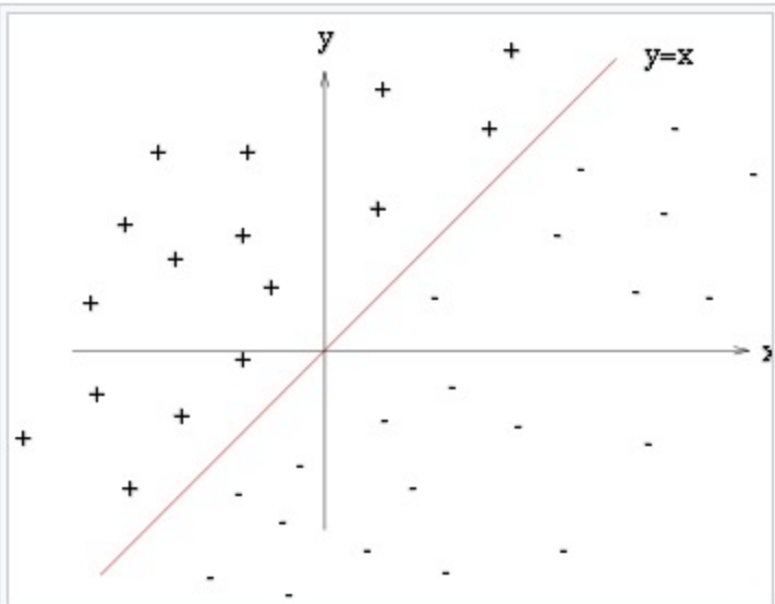
Exemple d'un problème de discrimination à deux classes, avec une séparatrice linéaire : la droite d'équation y = x . Le problème est linéairement séparable .
