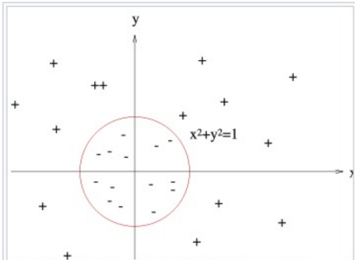
Exemple d'un problème de discrimination à deux classes, avec une séparatrice non-linéaire : le cercle unité . Le problème n'est pas linéairement séparable .
