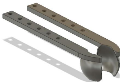
Modèle 3D de l'embout de la pince pour saisir les balles
