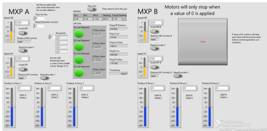
Exemple d'un visuel de panneau de contrôle permettant de tester les capteurs et les actionneurs
