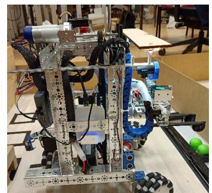
Système lève palette
