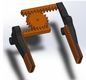
Principe mécanique de la pince
