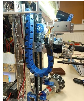
Chaîne passe câbles
