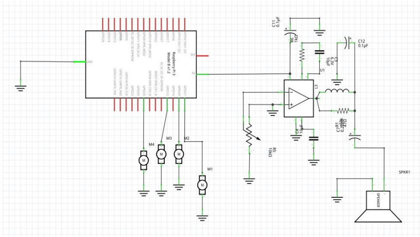
Fig13: schématique sur fritzing
