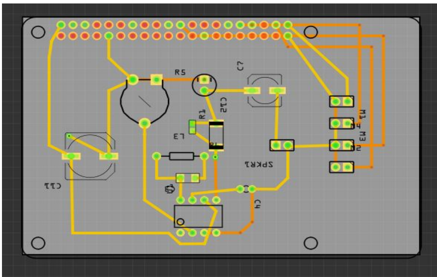
Fig14: pcb sur fritzing
